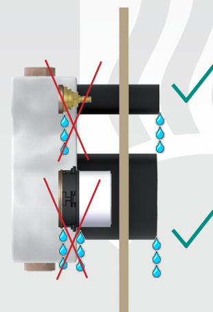
bei Ventil und Wasserzähler kein Tropfwasser in der Wand möglich
