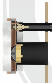
Aufbau Tropfschutzkappen
